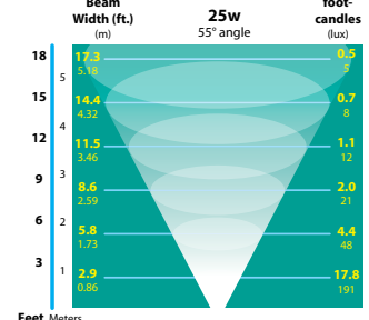
25w PAR36 (VWFL)
